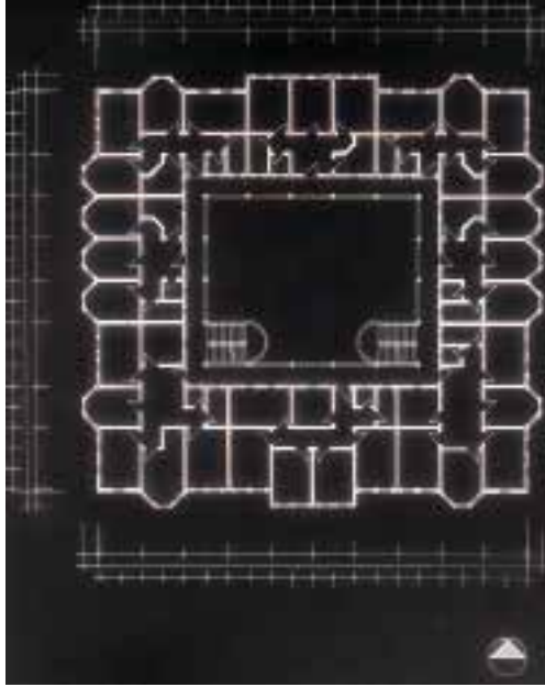
Resim 44. İstanbul-Laleli: Harikzedegan Apartmanları, tip kat planı. (Y. Yavuz)
