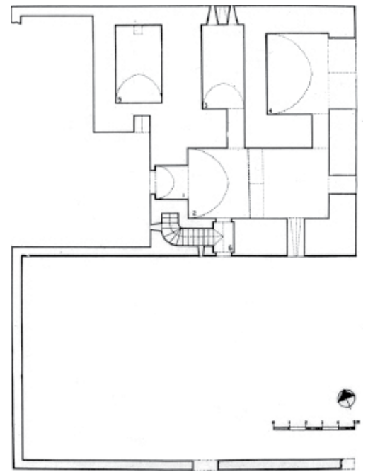
Resim 23. Alanya-Demirtaş: Syedre Kasrı alt kat planı. (Y. Yavuz)
