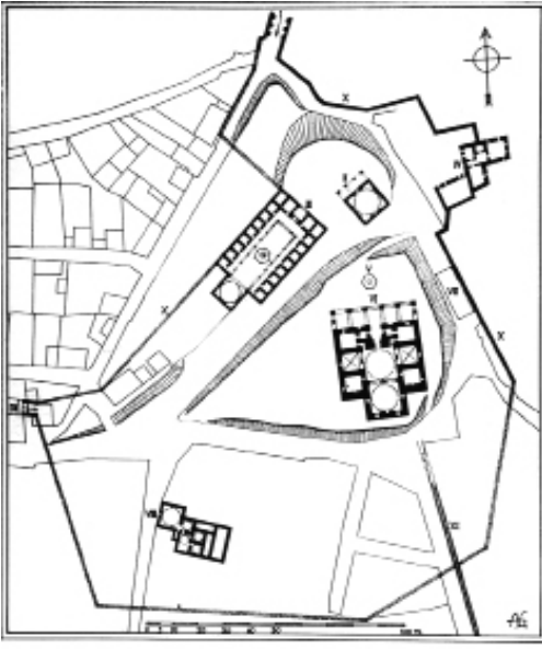
Resim 24. Bursa: kale planı, 15 yy. (A. Gabriel).
