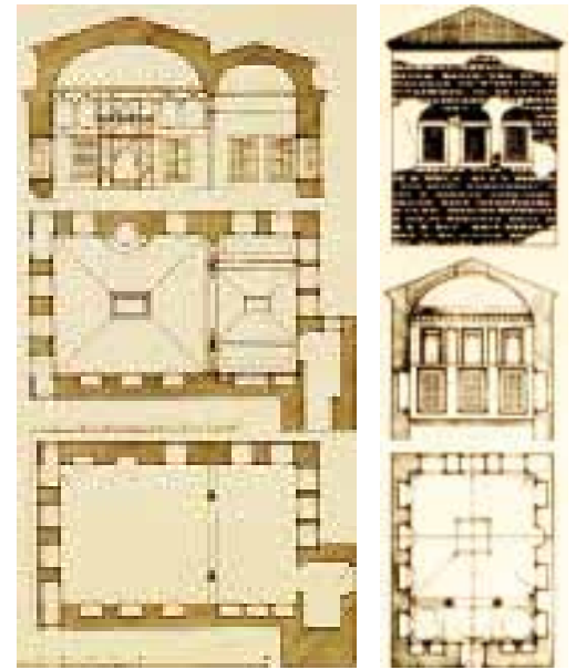
Resim 20. İstanbul-Fener'de tek odalı ev planı. (Y. Sey - U. Tanyeli)
