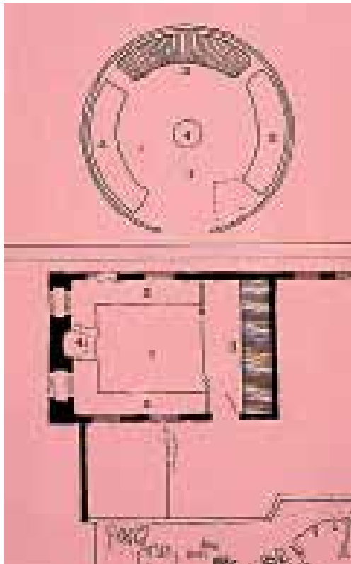
Resim 15. Orta Asya tipi yurt planı ve Anadolu tipi Türk odası planı. (Ö. Küçükerman)
