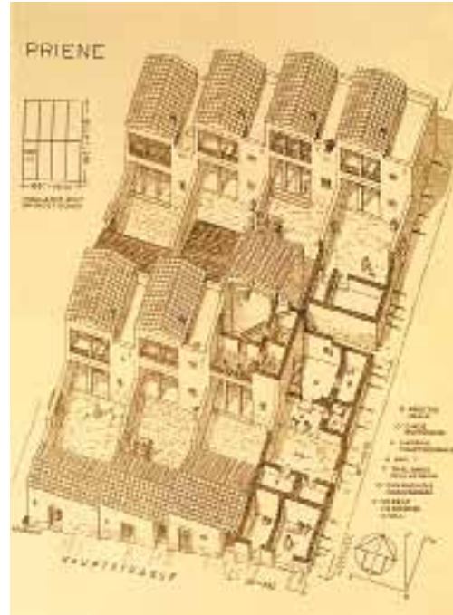
Resim 22. Priene: Prostos-oikos tipi sıra evler (restitüsyon). (Y. Sey - Haluk Abbasoğlu)
