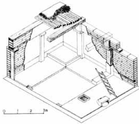
Resim 13. Çatalhöyük: Tek konut analizi (restitüsyon). (J. Mellart)
