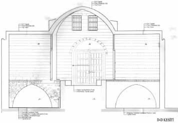
D-D Kesiti
