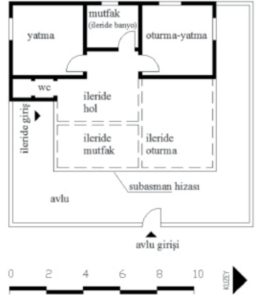
Resim 2. Dervişler mahallesi'ndeki konutun plan şeması.
